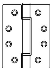
ANSI hole pattern
